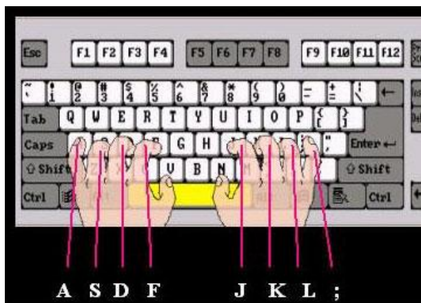
图 1-14 基本键位
