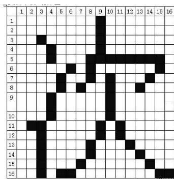
图 1-20 16 点阵字模
